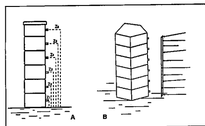
Fig. 2.- Esquema de las cajas primáticas. A: se presentan las diferentes alturas a las que se encuentran situadas los orificios de entrada de la nieve; en total la columna de cajas mide 1,5 m de altura. B: a partir de la masa recogida en las cajas se calcula la distribución vertical de flujo de nieve.
